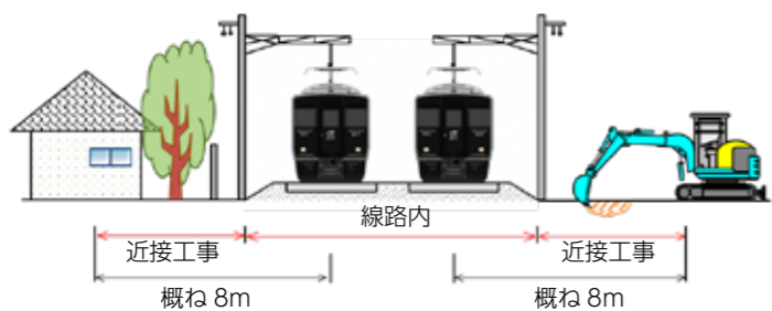
※作業内容や環境条件、使用重機によっては8m以上の場合でも近接工事の適用となる場合があります。
